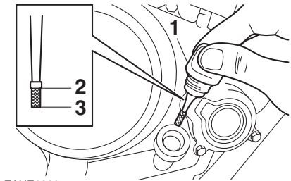
1. Tappo bocchettone riempimento olio motore
